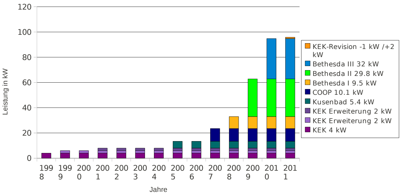
Zuwachs der einzelnen PV-Anlagen
